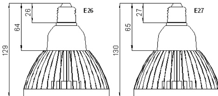
外形寸法
