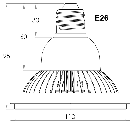
外形寸法
